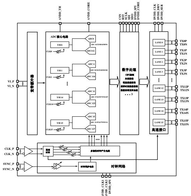
图 4-1 AAD08S020G 结构框图
